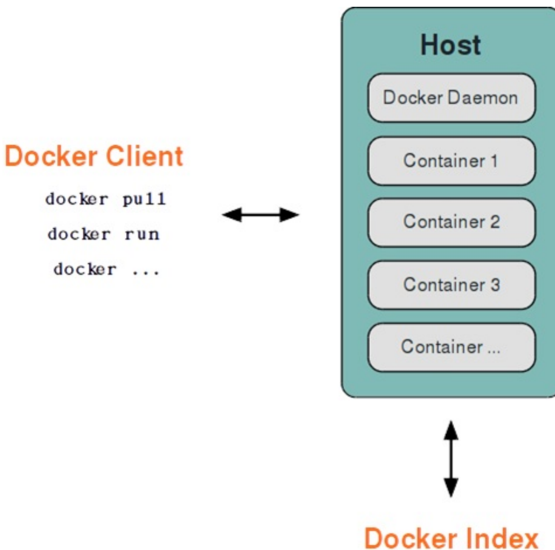
图 1.15.1.1 - Docker 基本架构
