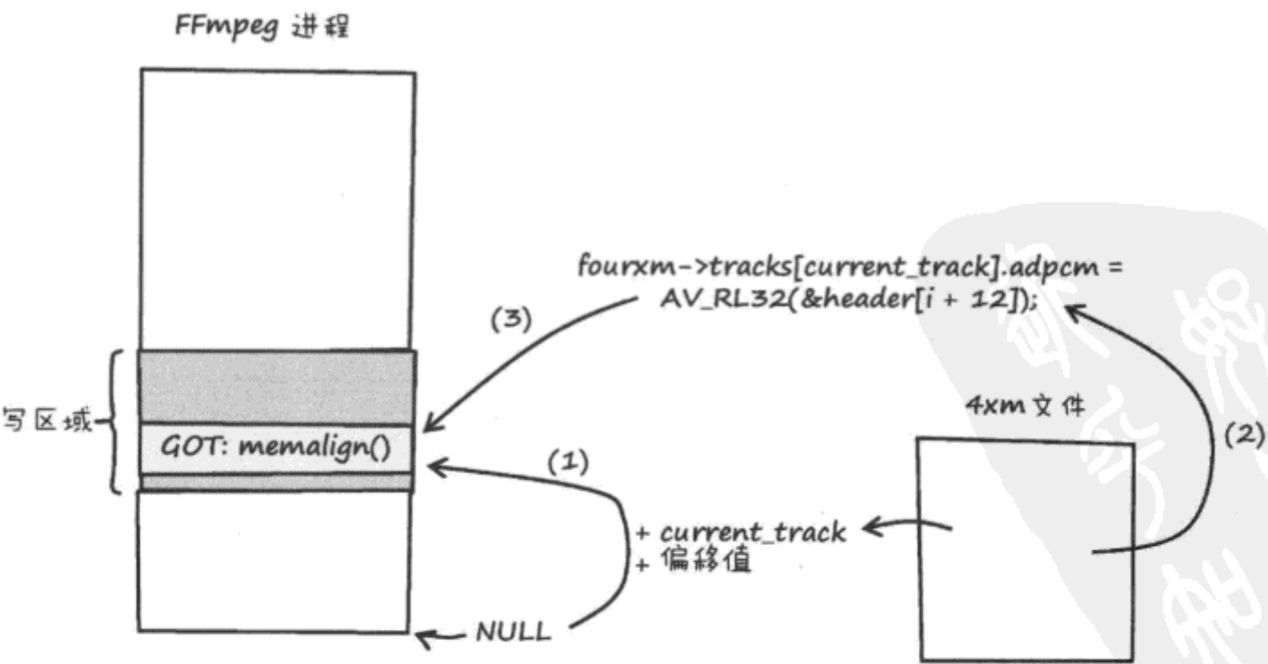
图 4-8 图解我是如何利用这个 FFmpeg bug 的
