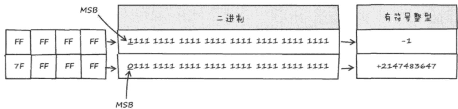
图 A-3 MSB 的作用
