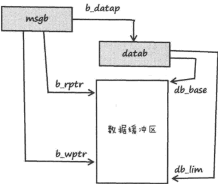
图 3-1 一个简单的 STREAMS 消息块
