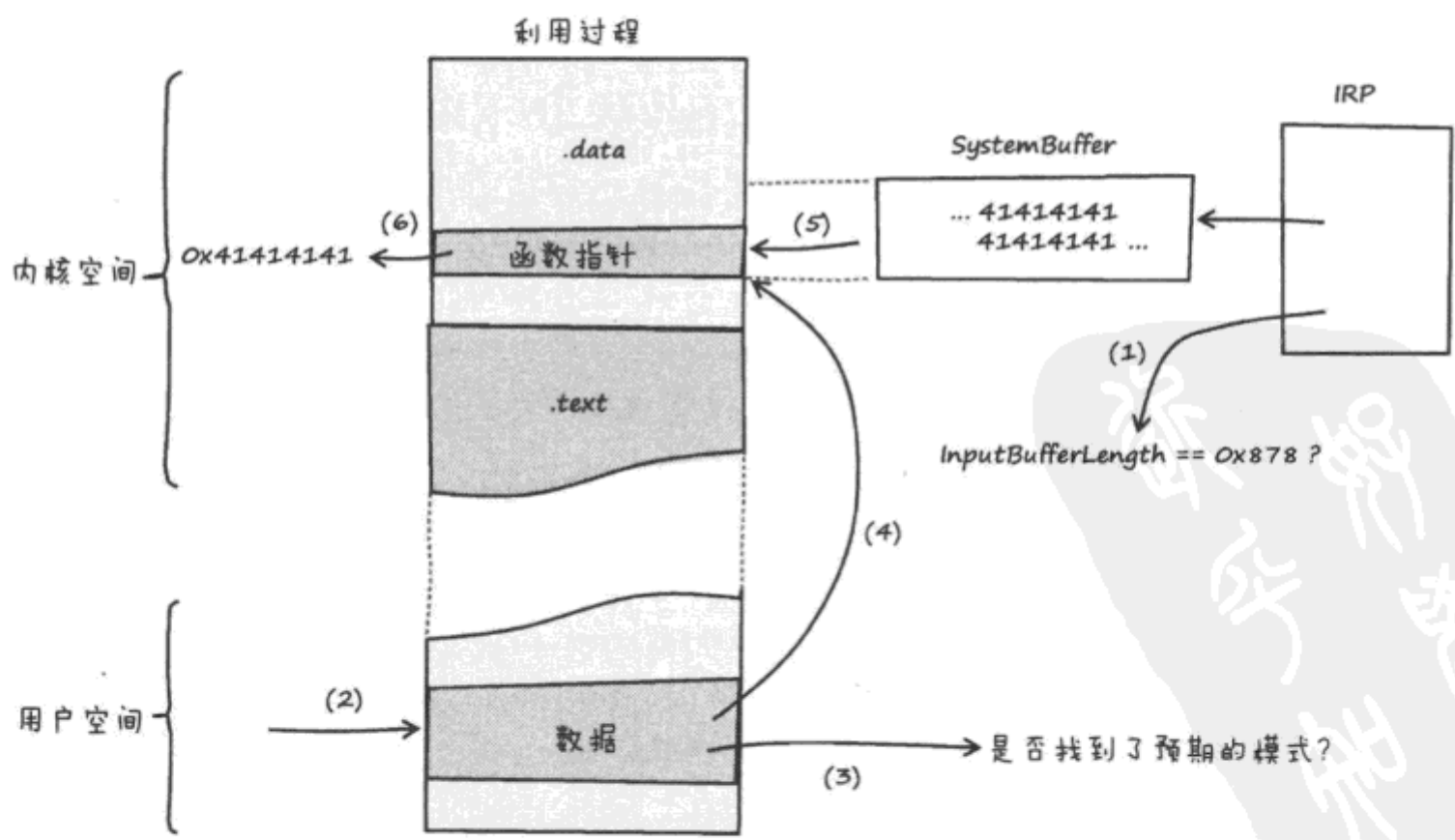
图 6-7 对 avast!漏洞的利用
