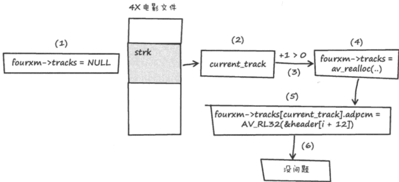
图 4-2 FFmpeg 正常运行时的期望行为
