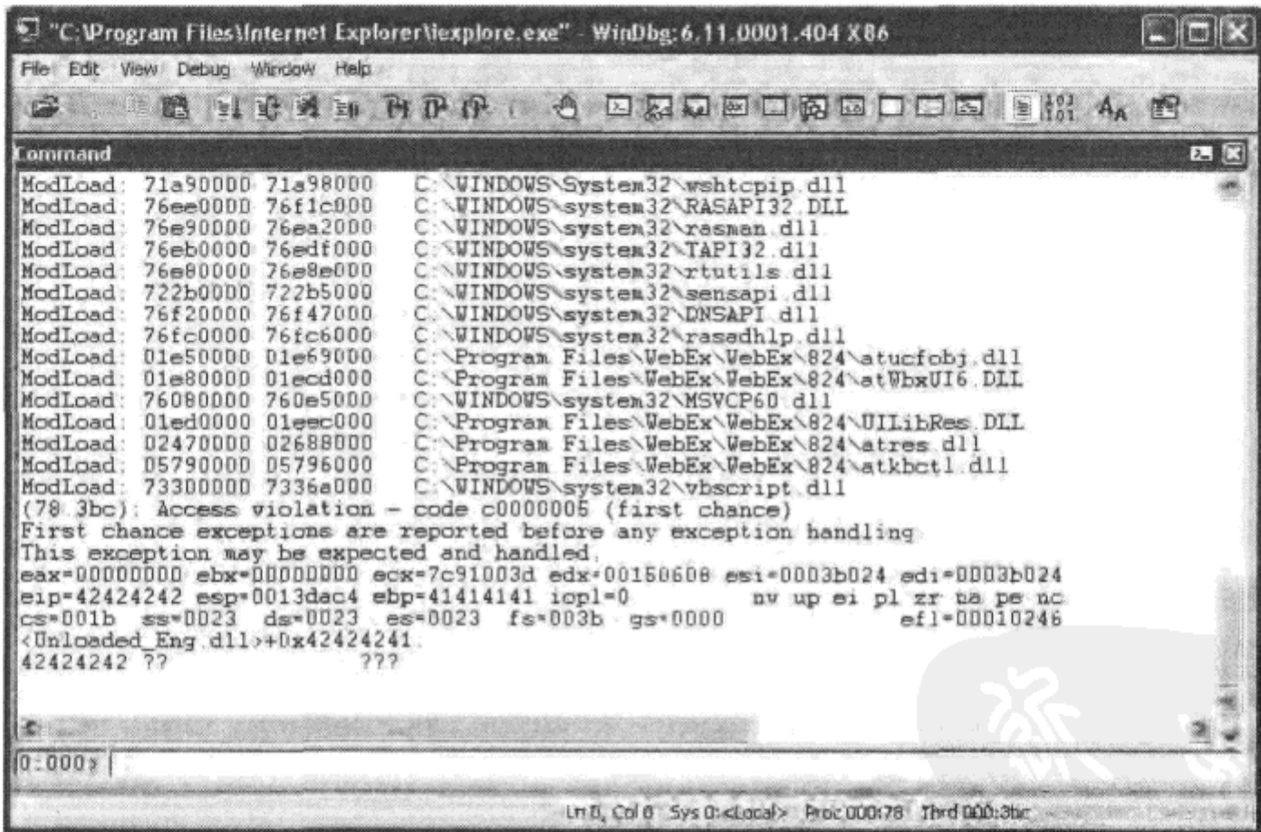
图 5-11 IE 的 EIP 控制
