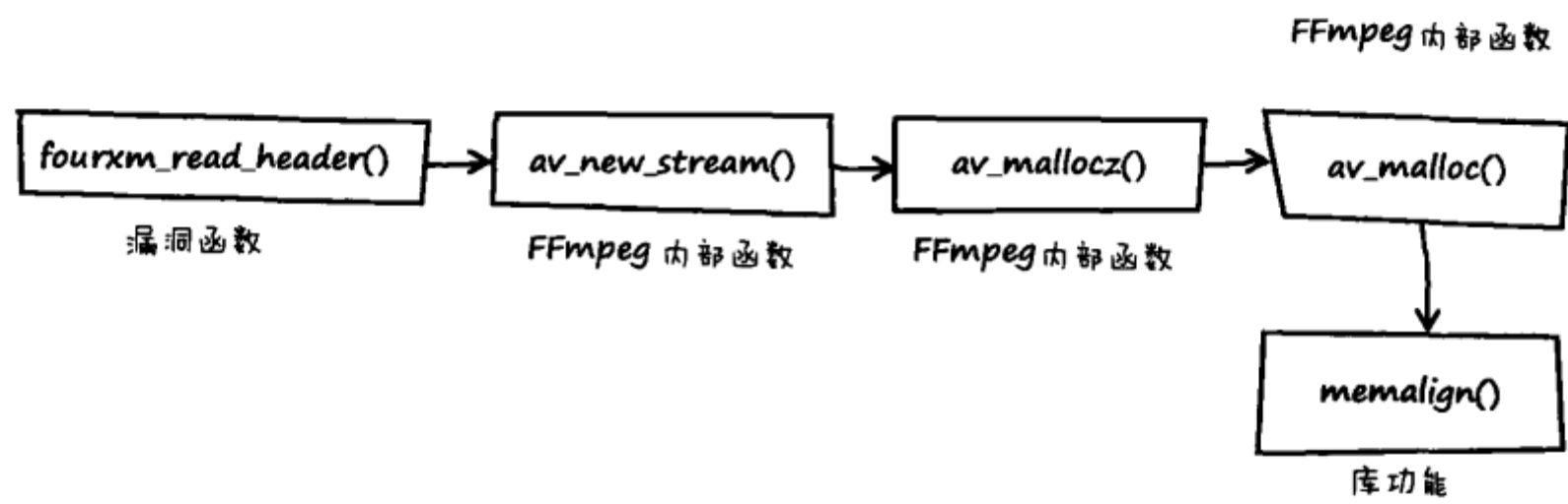
图 4-6 函数调用图,显示从漏洞函数到 memalign() 的调用关系
