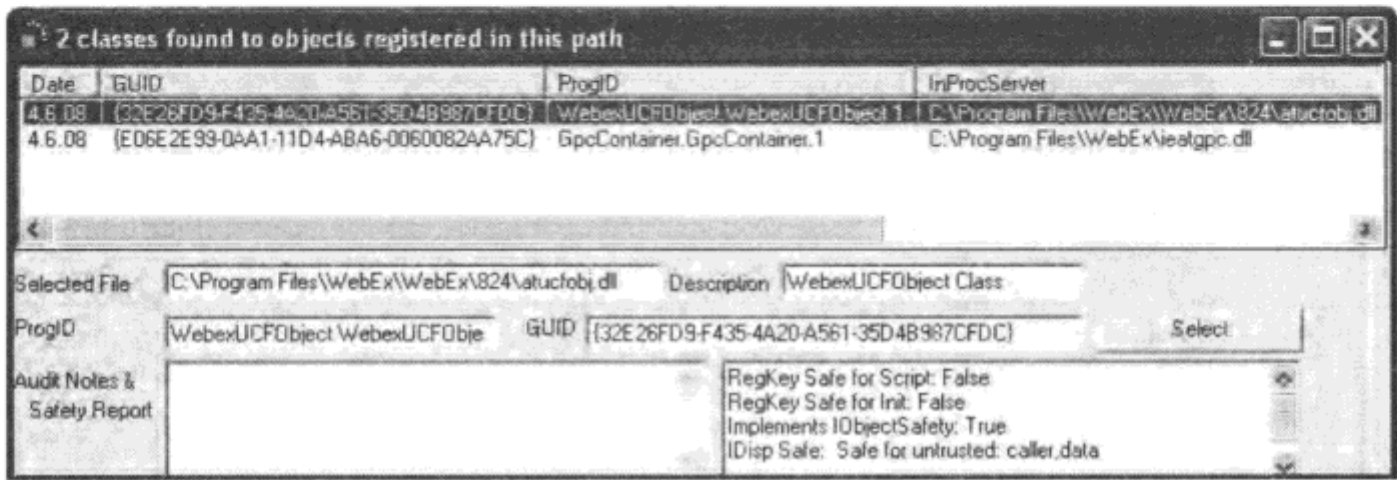
图 5-1 COMRaider 中 WebEx 注册的对象
