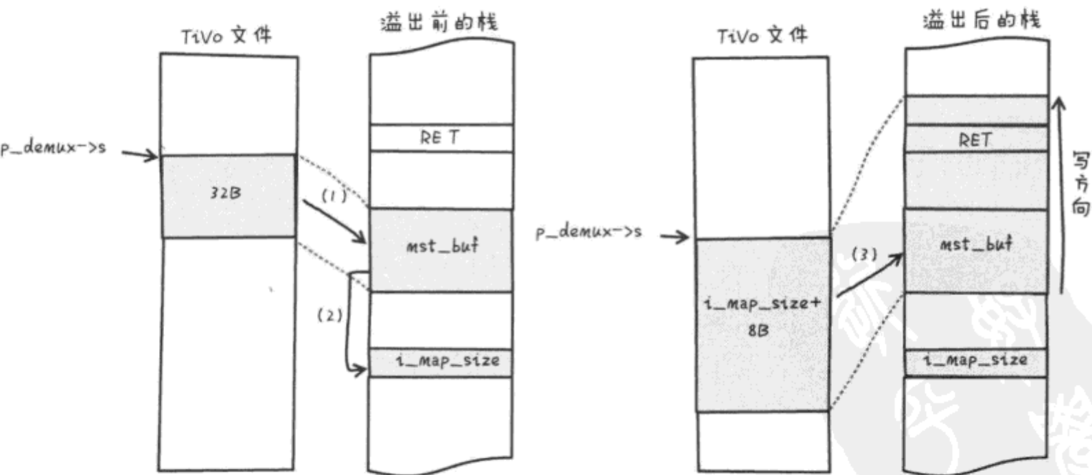
图 2-2 该漏洞从输入数据到栈缓冲区溢出的概览
