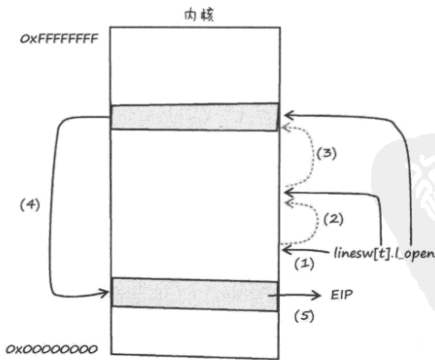
图 7-1 描绘我在 OS X 的 XNU 内核中发现的漏洞
