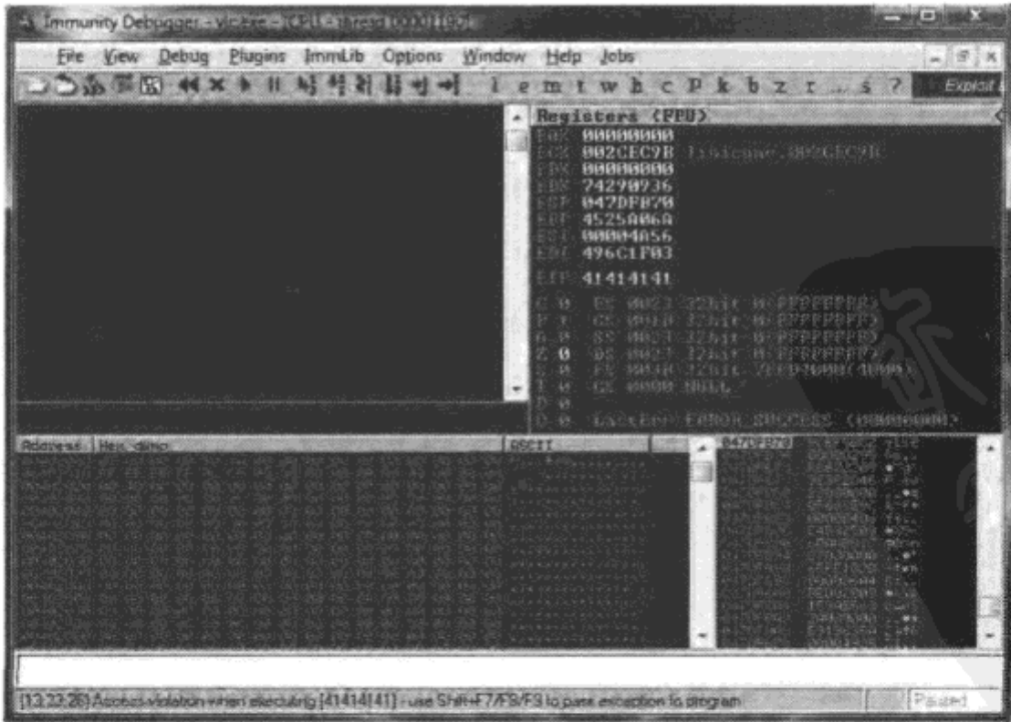
图 2-7 VLC 媒体播放器的 EIP 控制
