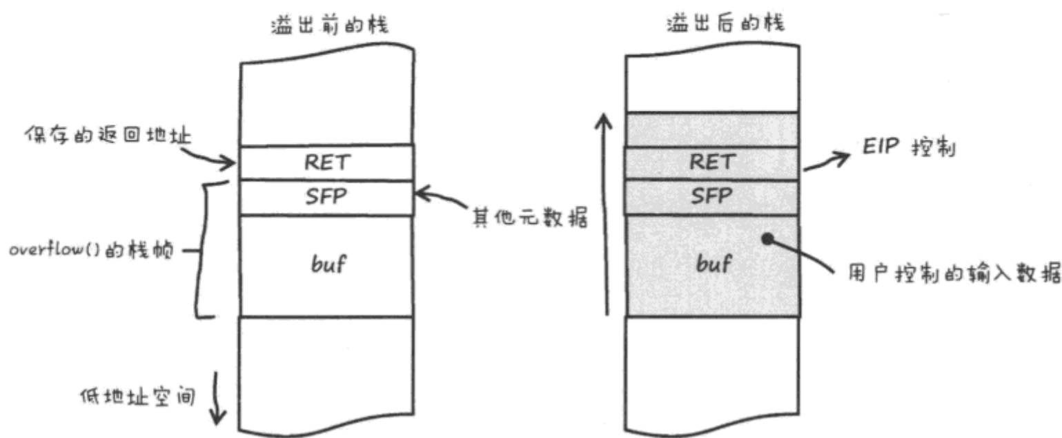
图 A-1 缓冲区溢出的栈帧布局
