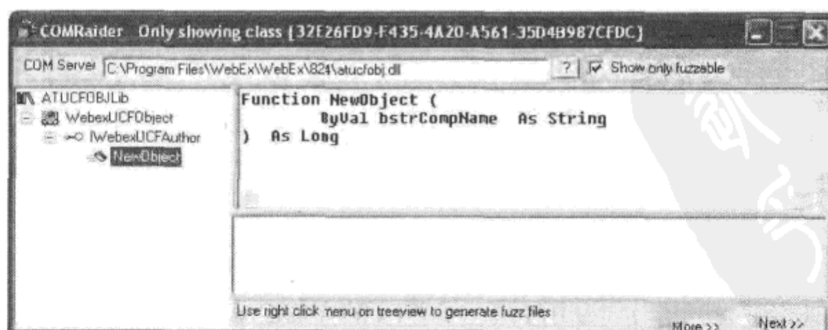
图 5-2 GUID 为{32E26FD9-F435-4A20-A561-35D4B987CFDC}的对象导出的公共方法
