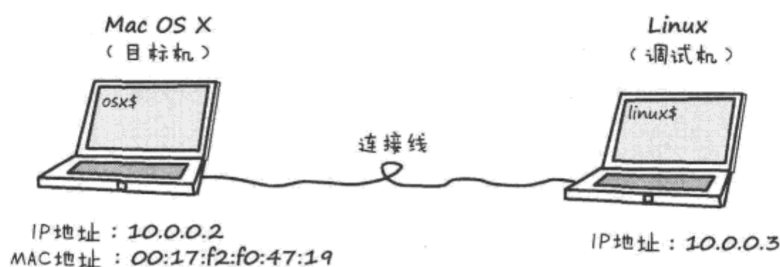
图 7-3 远程调试 Mac OS X 内核的装备
