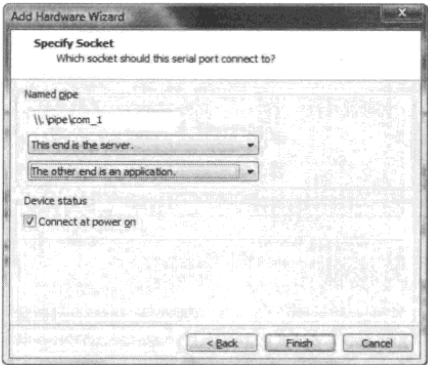
图 B-2 命名管道配置
