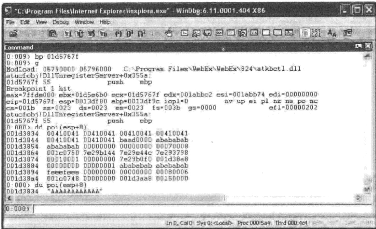
图 5-7 定义一个新的断点后 NewObject()函数的用户控制参数
