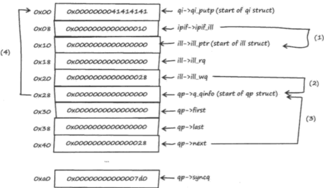
图 3-6 零页内存的数据布局
