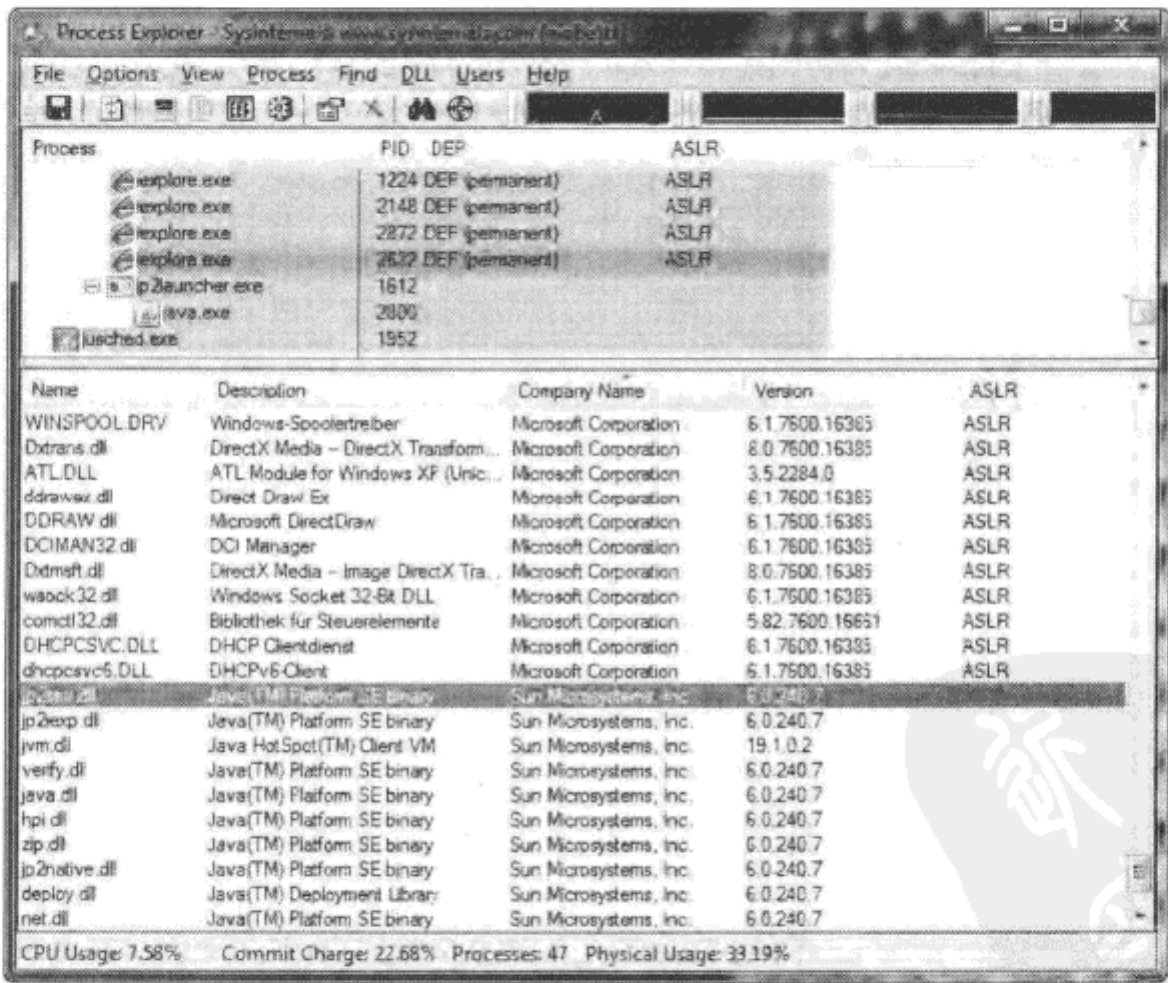
图 C-1 Process Explorer 中显示的 DEP 和 ASLR 状态
