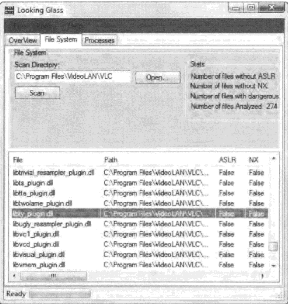
图 2-9 LookingGlass 扫描 VLC 的结果
