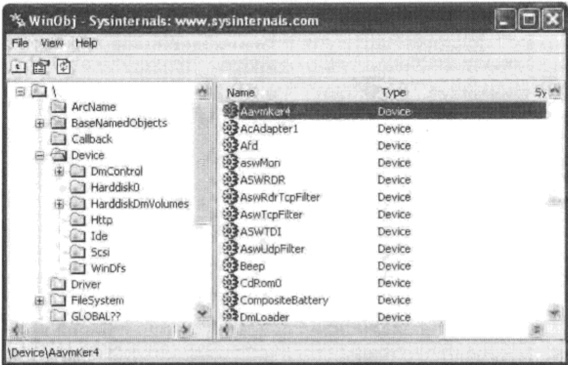
图 6-2 WinObj 中 AavmKer4 设备的安全设置导航
