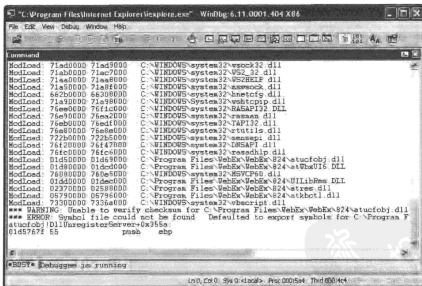
图 5-5 WinDbg 显示 NewObject() 方法的内存地址
