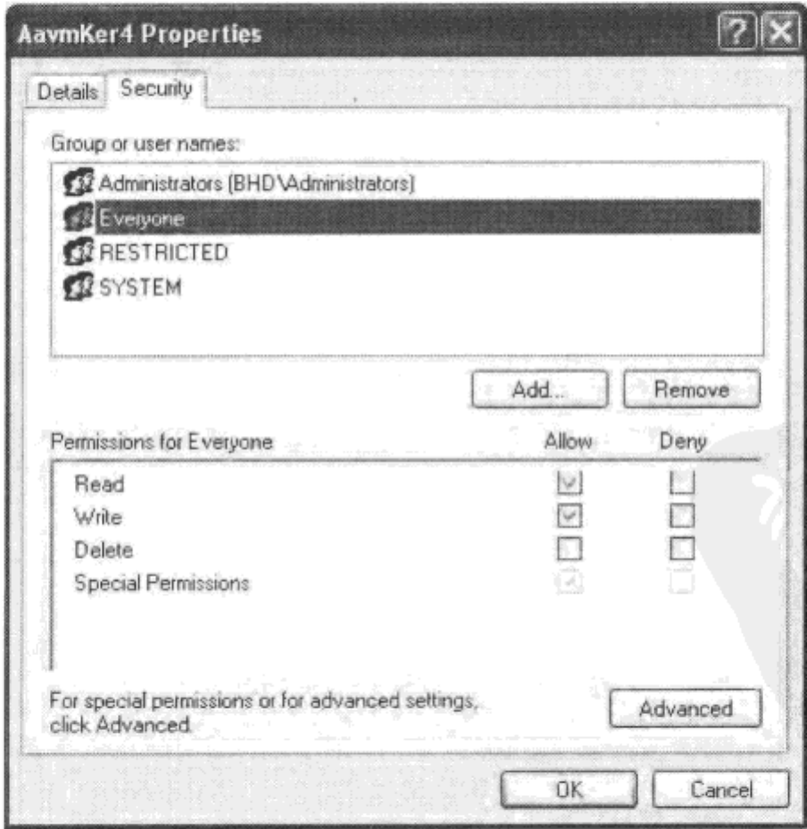
图 6-3 查看 \Device\AavmKer4 的安全设置
