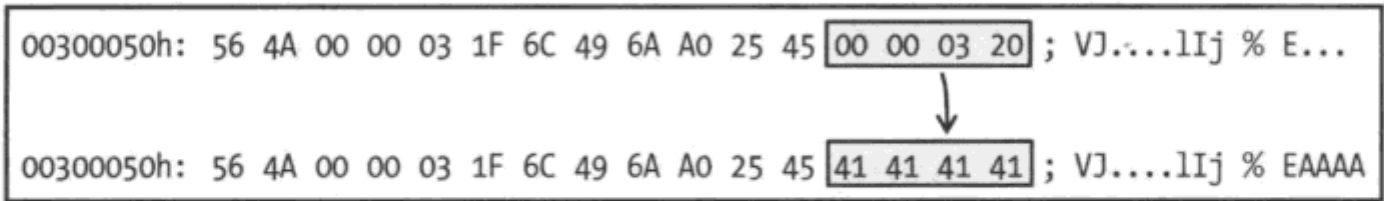
图 2-6 TiVo 样例文件中 EIP 的新值
