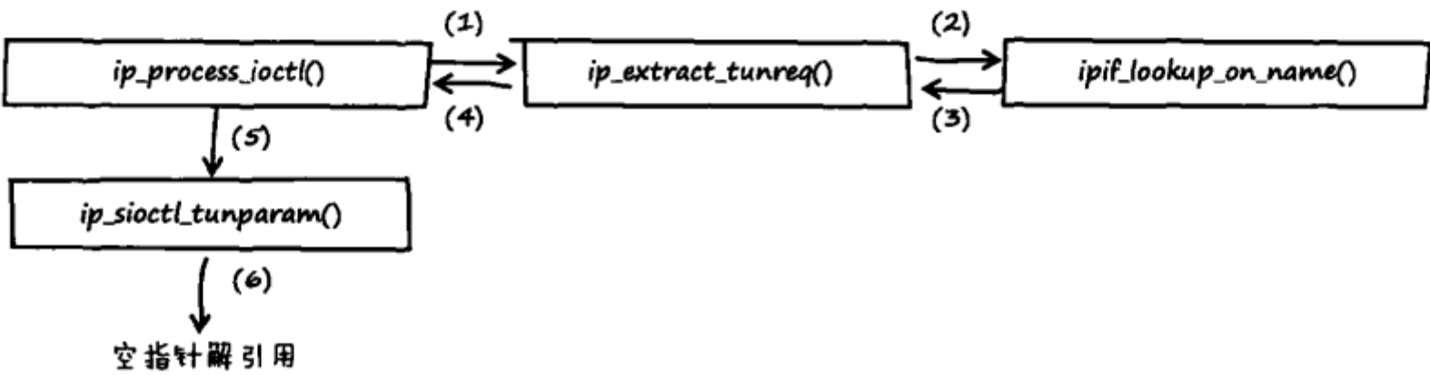
图 3-4 调用图总结空指针解引用 bug 涉及的函数调用关系。数字指事件的时间顺序
