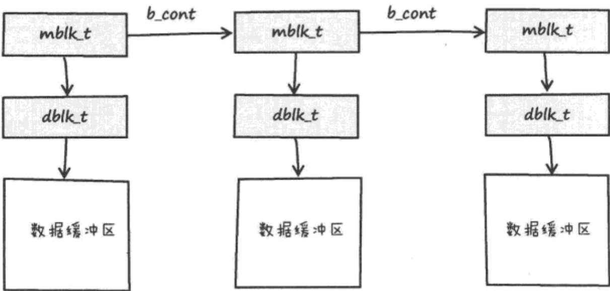
图 3-2 链接的 STREAMS 消息块
