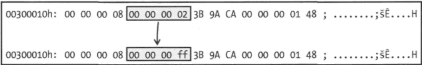
图 2-4 TiVo 样例文件中 i_map_size 的新值
