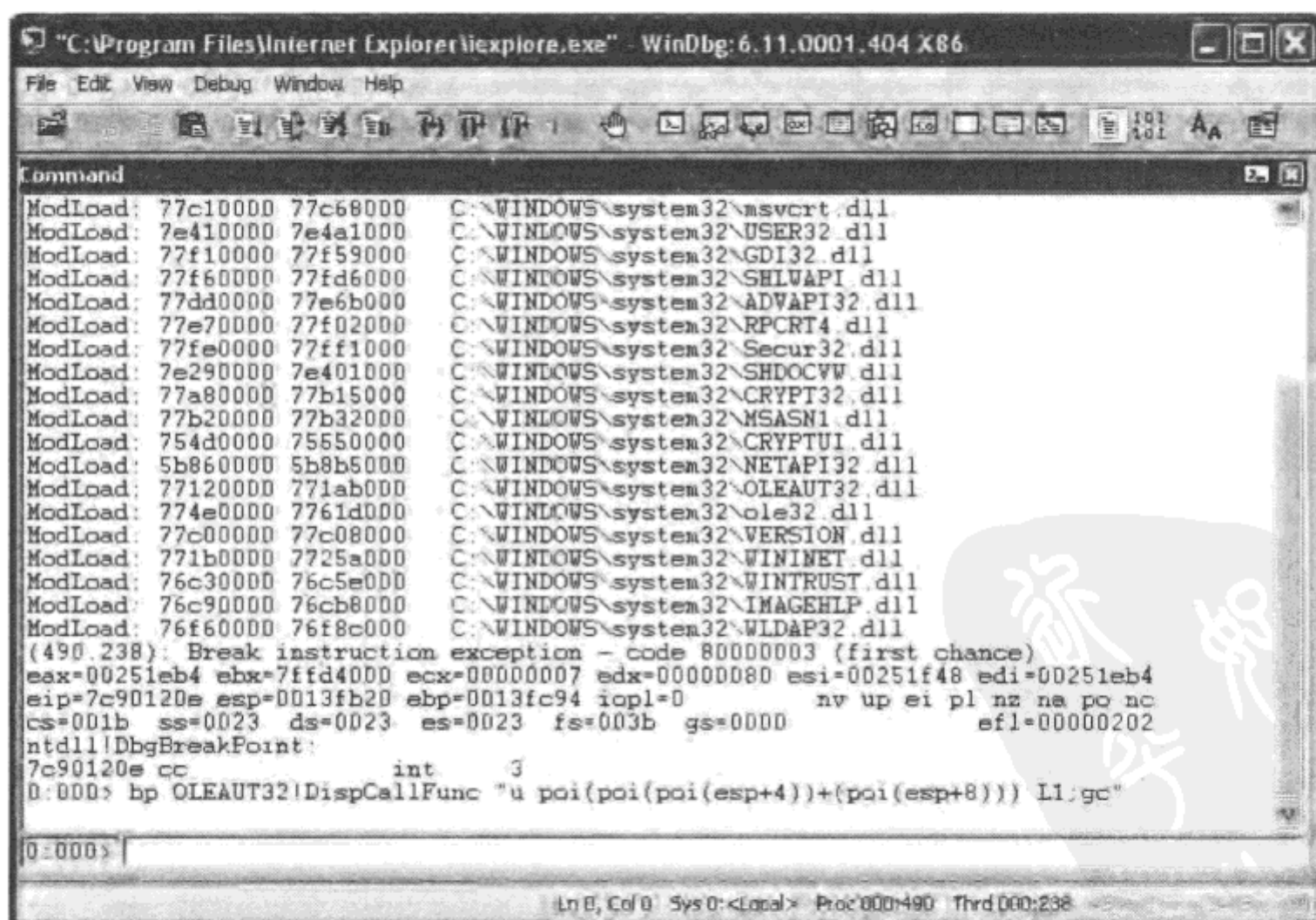
图 5-4 在 IE 中的 OLEAUT32!DispCallFunc 处定义一个断点
