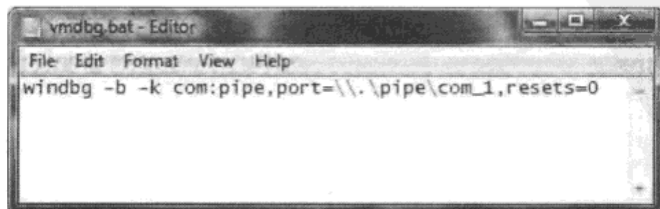
图 B-5 内核调试用的 WinDbg 批处理文件
