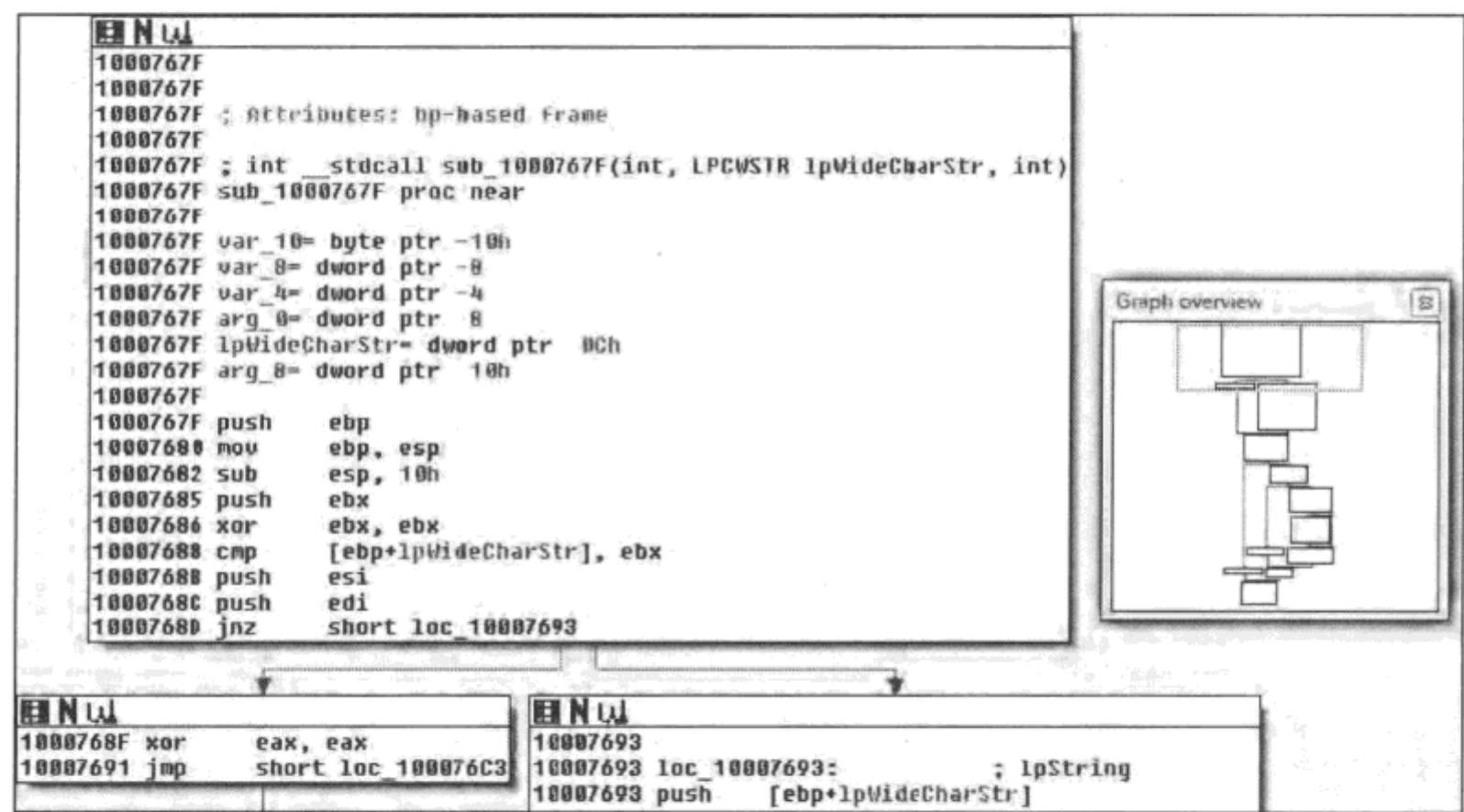
图 5-6 IDA Pro 中反汇编 NewObject() 方法
