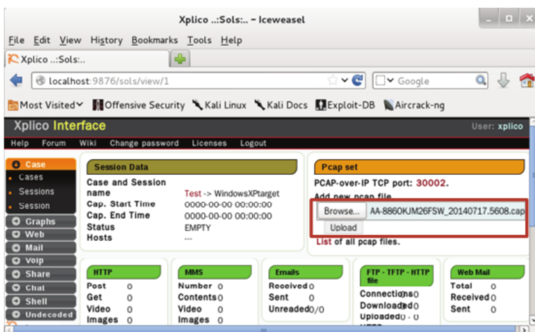
图 6.27 上传 pcap 文件
