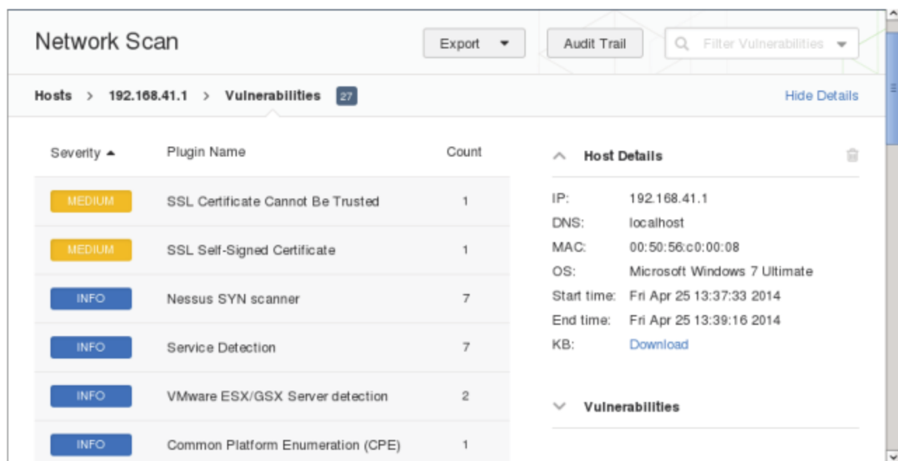
图 5.25 网络扫描结果
