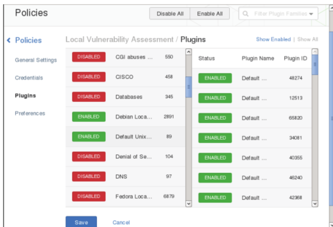
图 5.13 启动的插件程序
