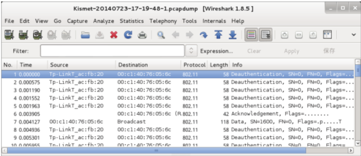
图 9.12 pcapdump 文件数据包
