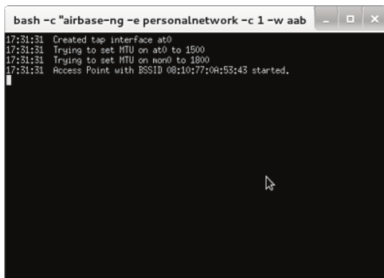
图 9.33 启动假接入点
