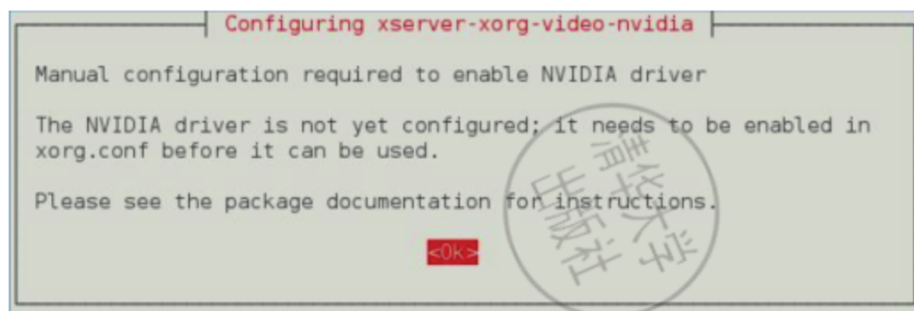
图 2.1 配置 xserver-xorg
