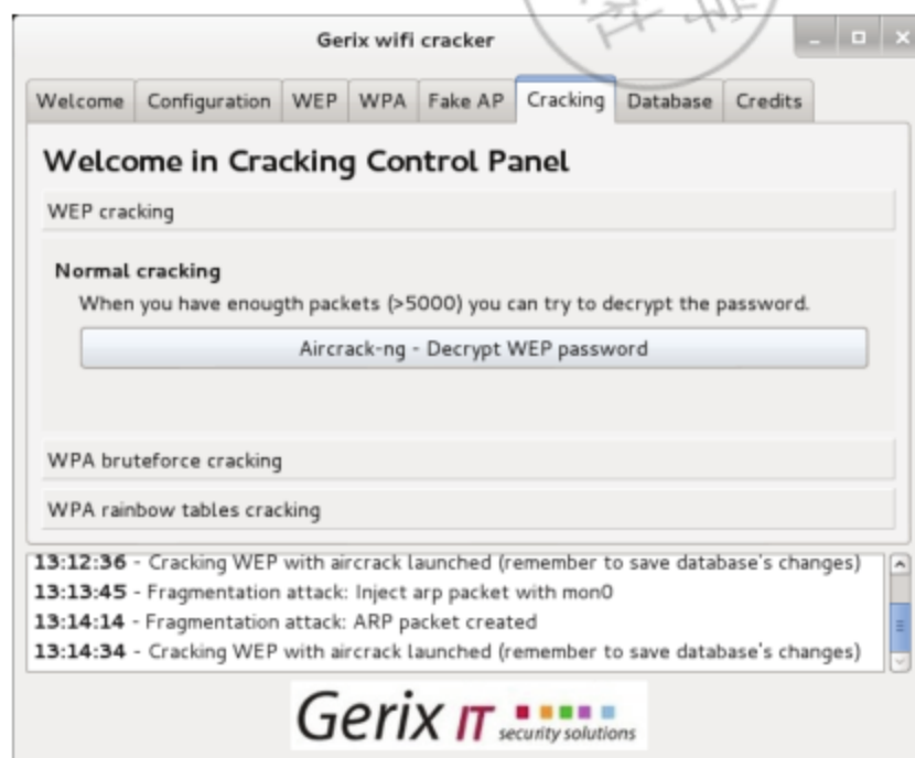
图 9.29 破解 WEP 密码
