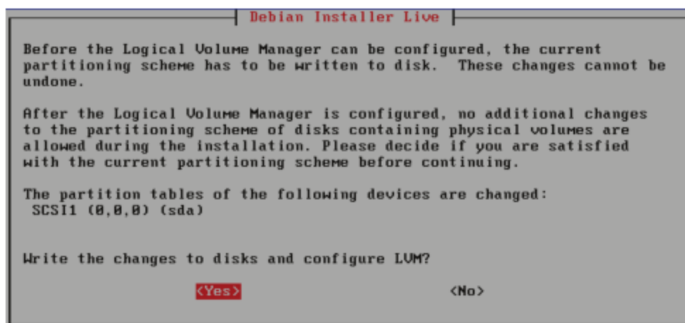
图 3.15 将数据写入磁盘
