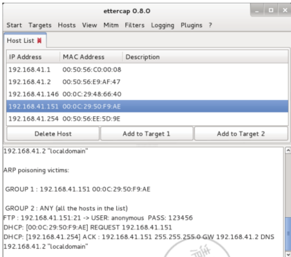
图 7.17 捕获到的敏感信息
