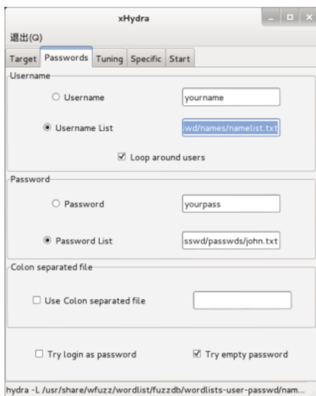
图 8.2 指定密码字典
