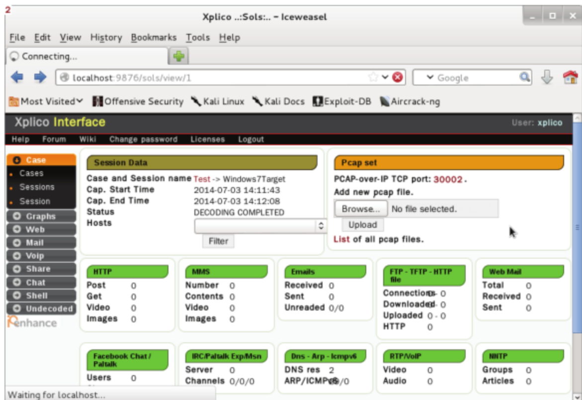
图 6.28 成功上传了捕获文件
