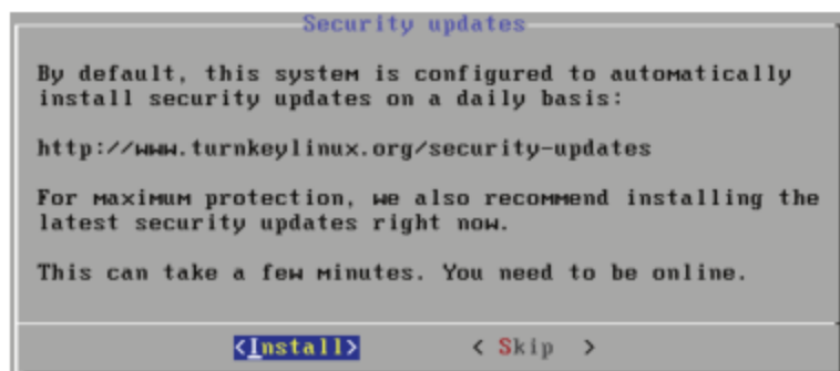
图 3.30 Security updates
